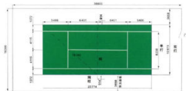
标准网球场尺寸图 (单位: 毫米)
