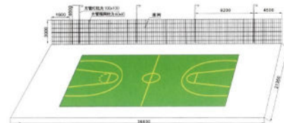
标准篮球场围网结构图 (单位: 毫米)
