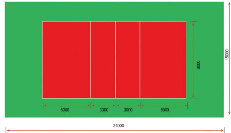
笼式排球场标准平面图
