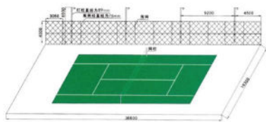
标准网球场围网结构图 (单位: 毫米)
