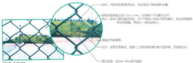
网球场围网
