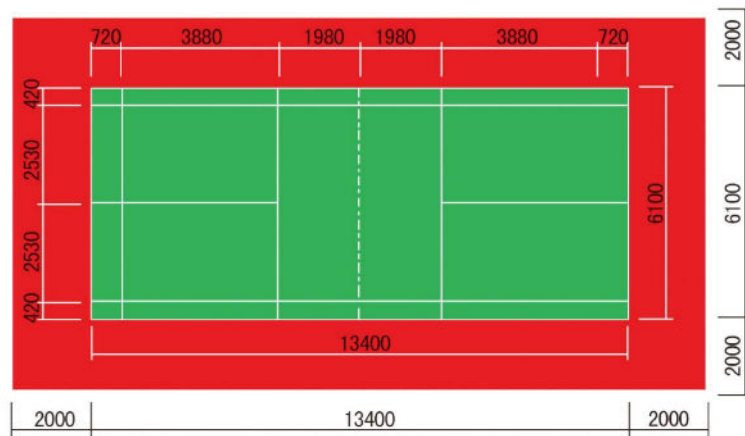
笼式羽毛球场标准平面图
