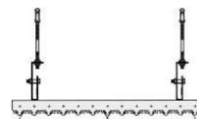
斜角条扣拼装示意图
