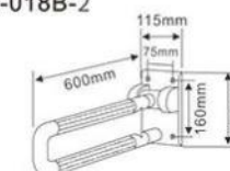
HS-018B-2
