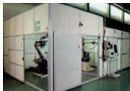
雷射和接机 X1 (1000W 德国制) Laser Welding Machine
