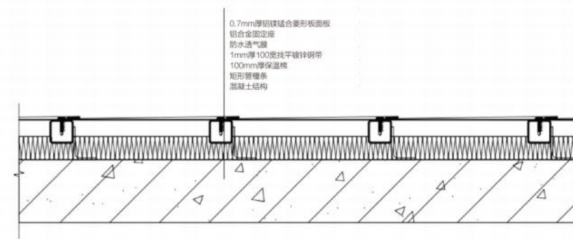
横剖面
