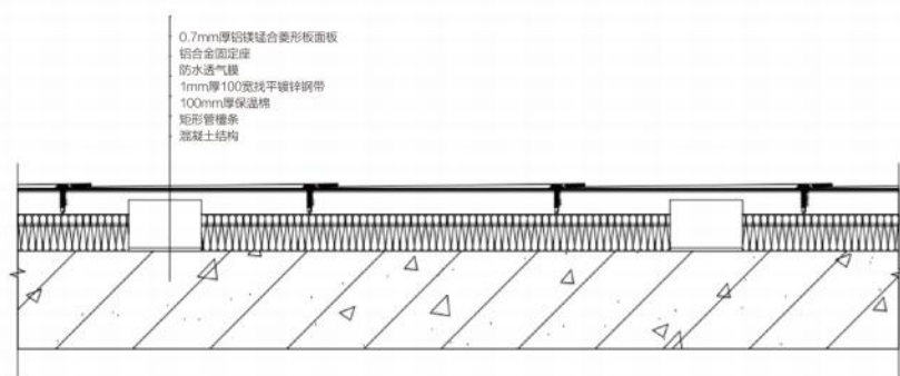
竖剖面
