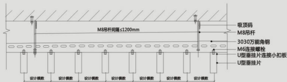
U型挂片横向剖面
