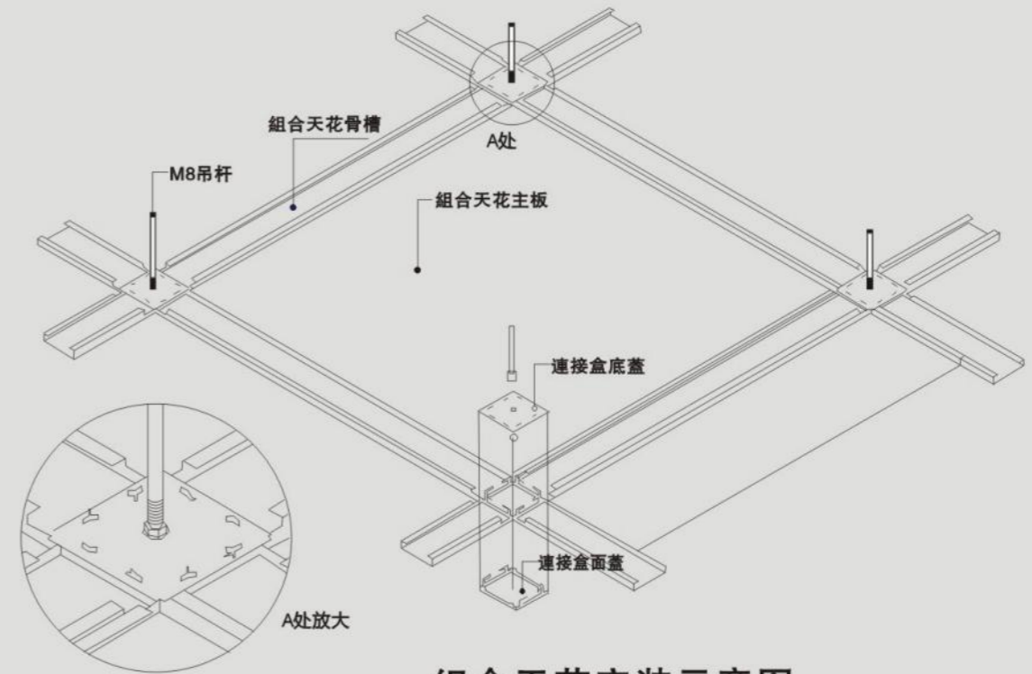
组合天花安装示意图
