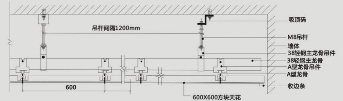
暗架式天花结构横向剖面图
