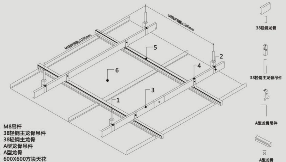
方板暗架式结构安装图
