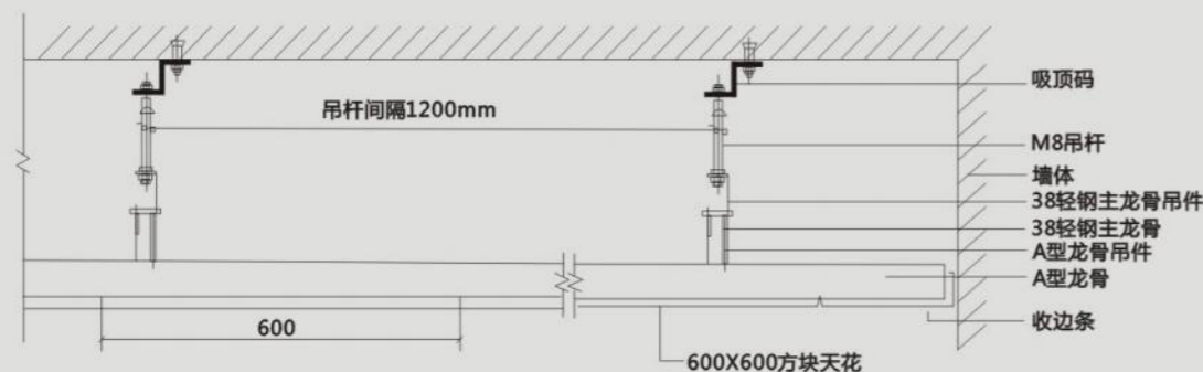
暗架式天花结构纵向剖面图
