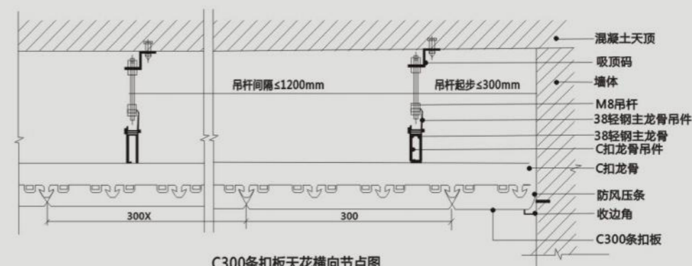
C300条扣板天花横向节点图
