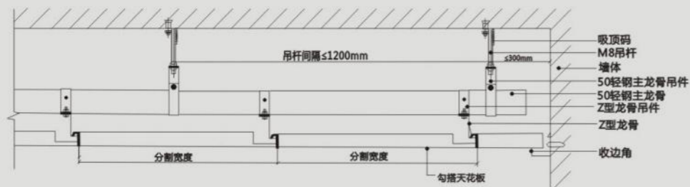
勾搭天花横向剖面
