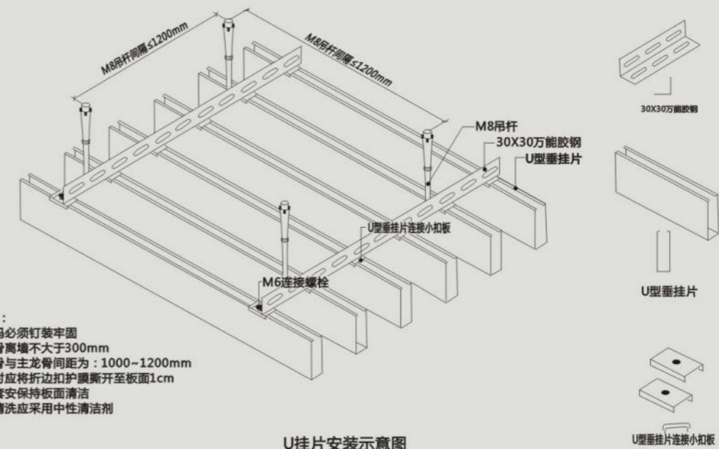
U挂片安装示意图
