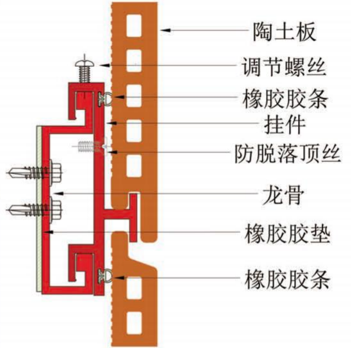
高层防坠
