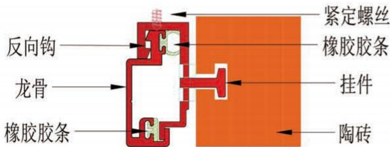
方砖反向钩挂件
