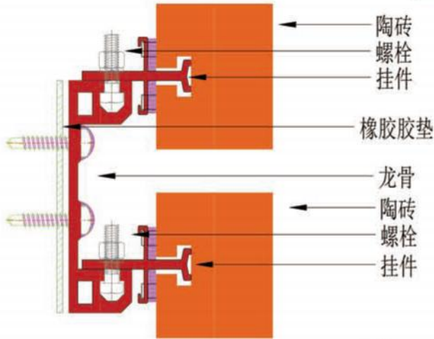
方砖螺栓干挂
