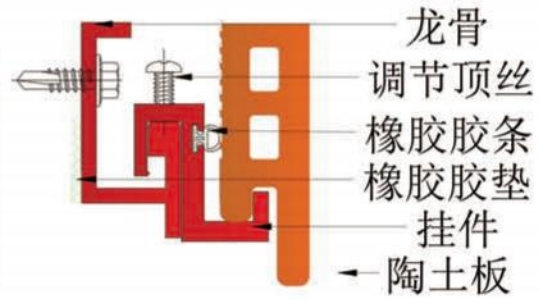
高层防坠—底收口
