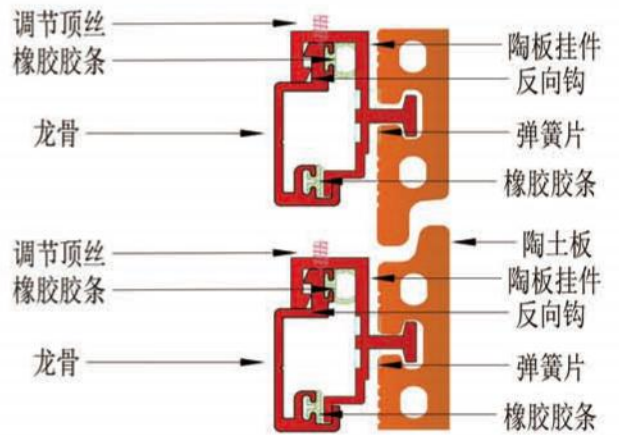
陶板背栓系统 (02)
