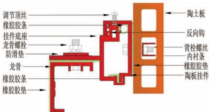
陶板背栓系统 (03)
