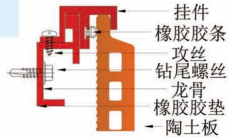
高层防坠—上收口
