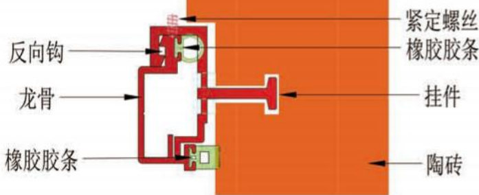
方砖反向钩防坠系统
