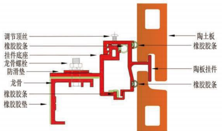
陶板背栓系统 (04)
