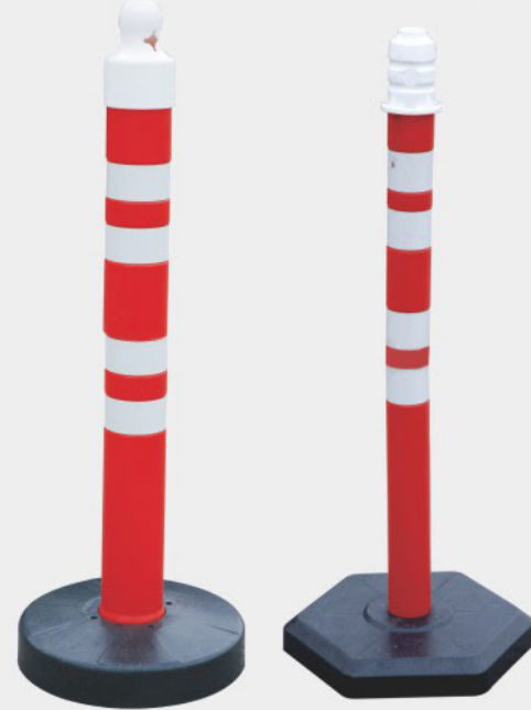
高度: 1150mmX120mm 重量: 3kgs 高度: 1000mmX60mm 重量: 1.8kgs
