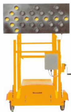
太阳能工程指示车 (小车) 指示屏尺寸: 1200×600 1400×600 灯筒尺寸: φ175
