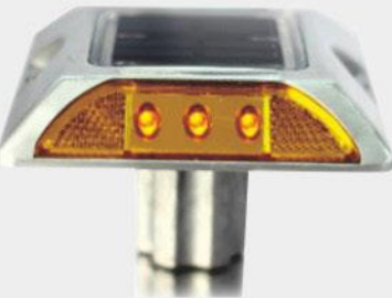
型号(model):LZL-DD-06 材料(material):铝(aluminium); 太阳能电池(solar battery) 尺寸(size):130x118MM
