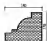
EPS-34 规格: 340 X 270
