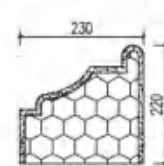
EPS-41 规格: 220 X 230
