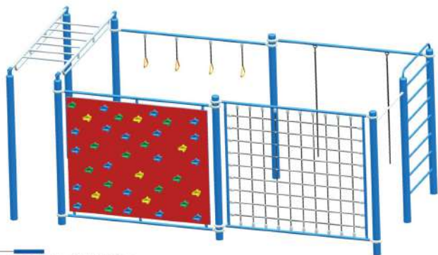
YATZH-001 综合训练器 1 规格: 6000x3000x2300mm
