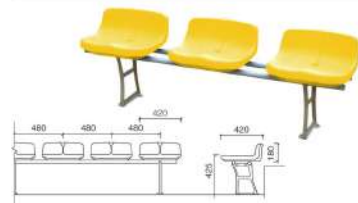
YATXJ-006 直立式中空塑料椅
